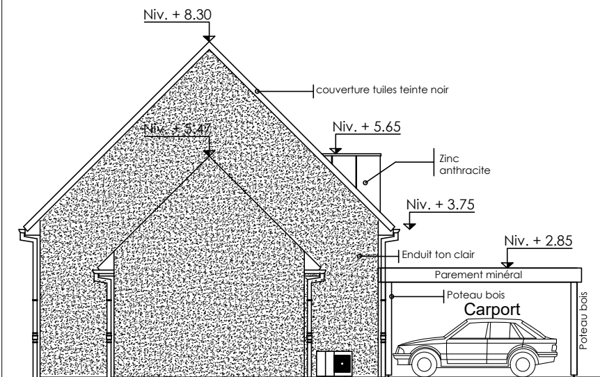
Pignon Gauche
