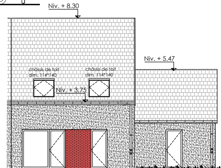
Façade Arrière
